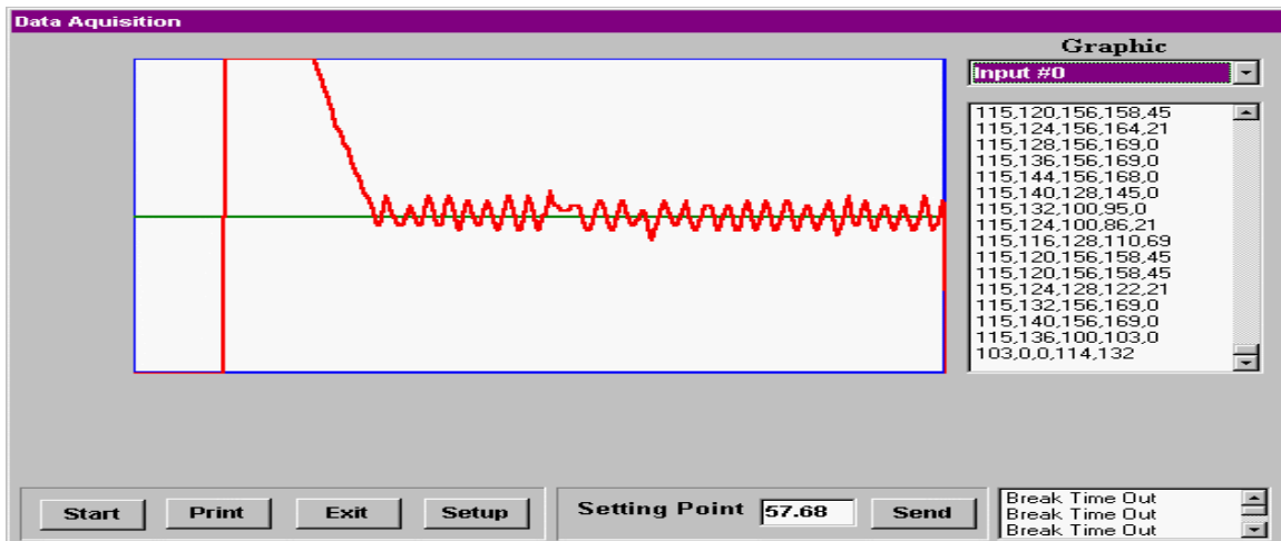
Gambar 16 Grafik Input Error
