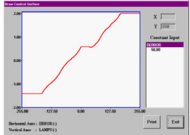
Gambar 11 Grafik Output Lampu terhadap Input Error dengan Delta_Error = 50
