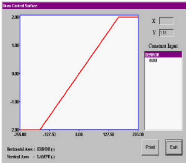
Gambar 10 Grafik Output Lampu terhadap Input Error dengan Delta_Error = 0
